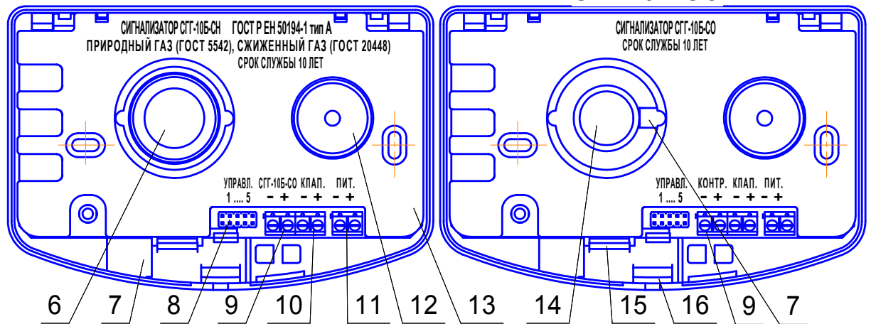
Вид спереди со снятой передней крышкой СГГ-10Б-СН
