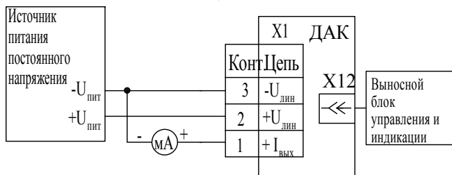
Схема электрическая подключений газоанализаторов к источнику питания
