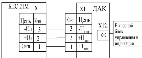
Схема электрическая подключений газоанализаторов к БПС-21М ИБЯЛ.411111.042, -01, -02, -05 ... -22
