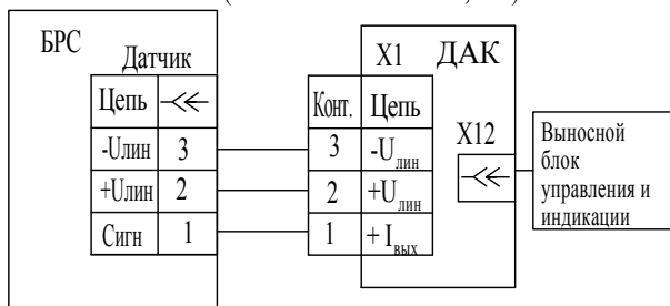
Схема электрическая подключений газоанализаторов к БРС (ИБЯЛ.411111.036-01, -02)
