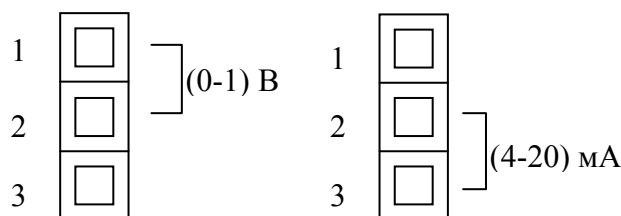
Рисунок 2.1 - Положение переключателей на кросс-плате для подключения выходного сигнала.
