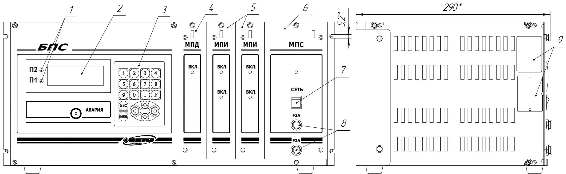
Вид сзади 480*
