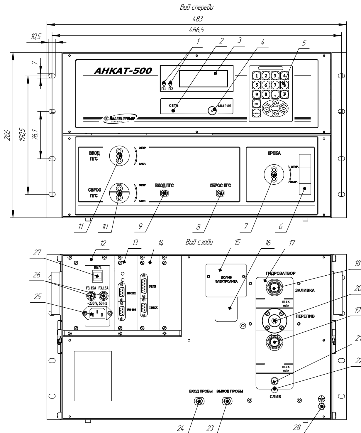
Рисунок 1.1 - Газоанализаторы АНКAТ-500. Внешний вид.
